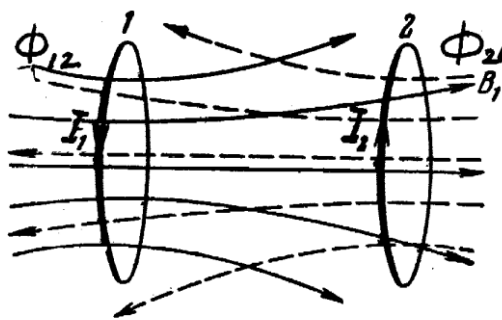
9.1-сурет. Екі контурдың өзара магниттік әсері.
